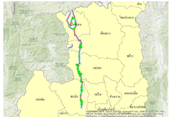
รูปที่ 5 รอยเลื่อนเวียงแหง
