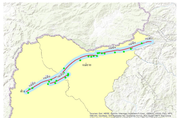
รูปที่ 7 รอยเลื่อนแม่จัน
