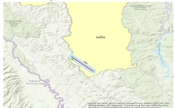
รูปที่ 6 รอยเลื่อนเมย
