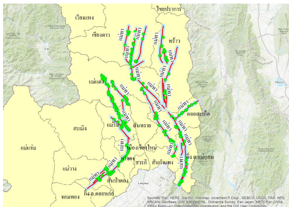
รูปที่ 4 รอยเลื่อนแม่ทา
