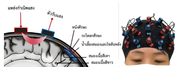
รูปที่ 3 หลักการทำงานของเทคนิคสเปกโทรสโกปีอินฟราเรด ย่านใกล้โดยใช้แหล่งกำเนิดแสงและตัวรับแสงในการตรวจวัดการเปลี่ยนแปลงความเข้มข้นของฮีโมโกลบินบริเวณเปลือกสมอง (ซ้าย) และตัวอย่างการติดตั้งอุปกรณ์ที่มีแหล่งกำเนิดแสงและตัวรับแสงสำหรับวัดกิจกรรมทางสมองบริเวณกลีบหน้าบนศีรษะของอาสาสมัคร (ขวา)
