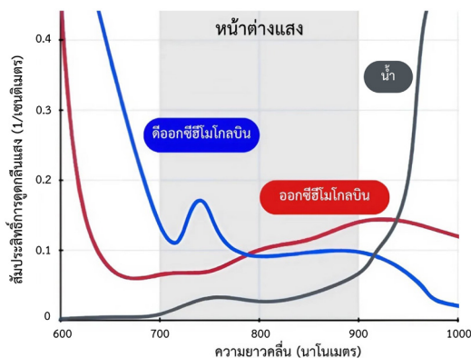
รูปที่ 2 การดูดกลืนแสงของออกซีโมโนโกลบิน ดีโออกซีโมโนโกลบิน และน้ำ ในช่วงคลื่นอินฟราเรดย่านใกล้ บริเวณแรงแสดงหน้าต่างแสง (Optical Window) ซึ่งเป็นช่วงคลื่นที่แสงสามารถทะลุผ่านเนื้อเยื่อได้ดี เหมาะสำหรับการวัดกิจกรรมสมองด้วยเทคนิคสเปกโทรสโกปีอินฟราเรดย่านใกล้
